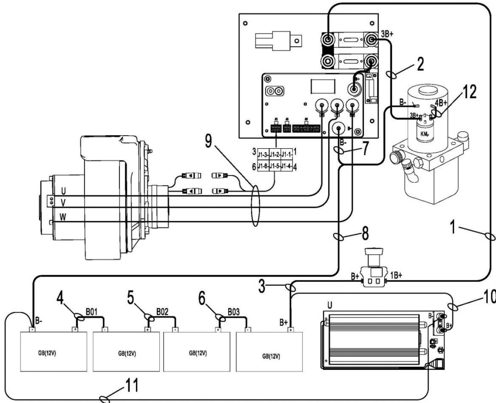
Fig. 20 Wiring Harness
